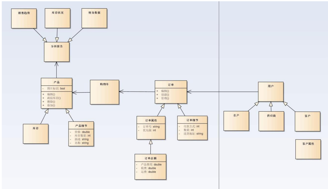
图三：类图
